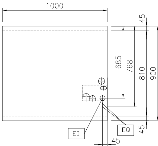
Boven aanzicht
